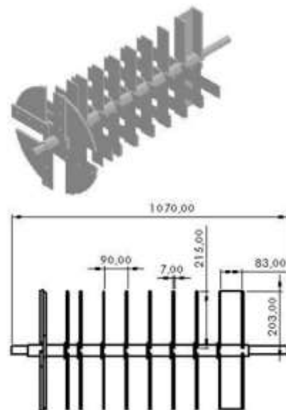
Gambar 2 Desain Mesin Pencacah Pelepah Sawit
